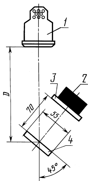
1 — ультрафиолетовый облучатель; 2 — датчик; 3 — светофильтр; 4 — люминесцентный экран
