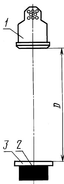
1 — ультрафиолетовый облучатель; 2 — датчик; 3 — светофильтр;
